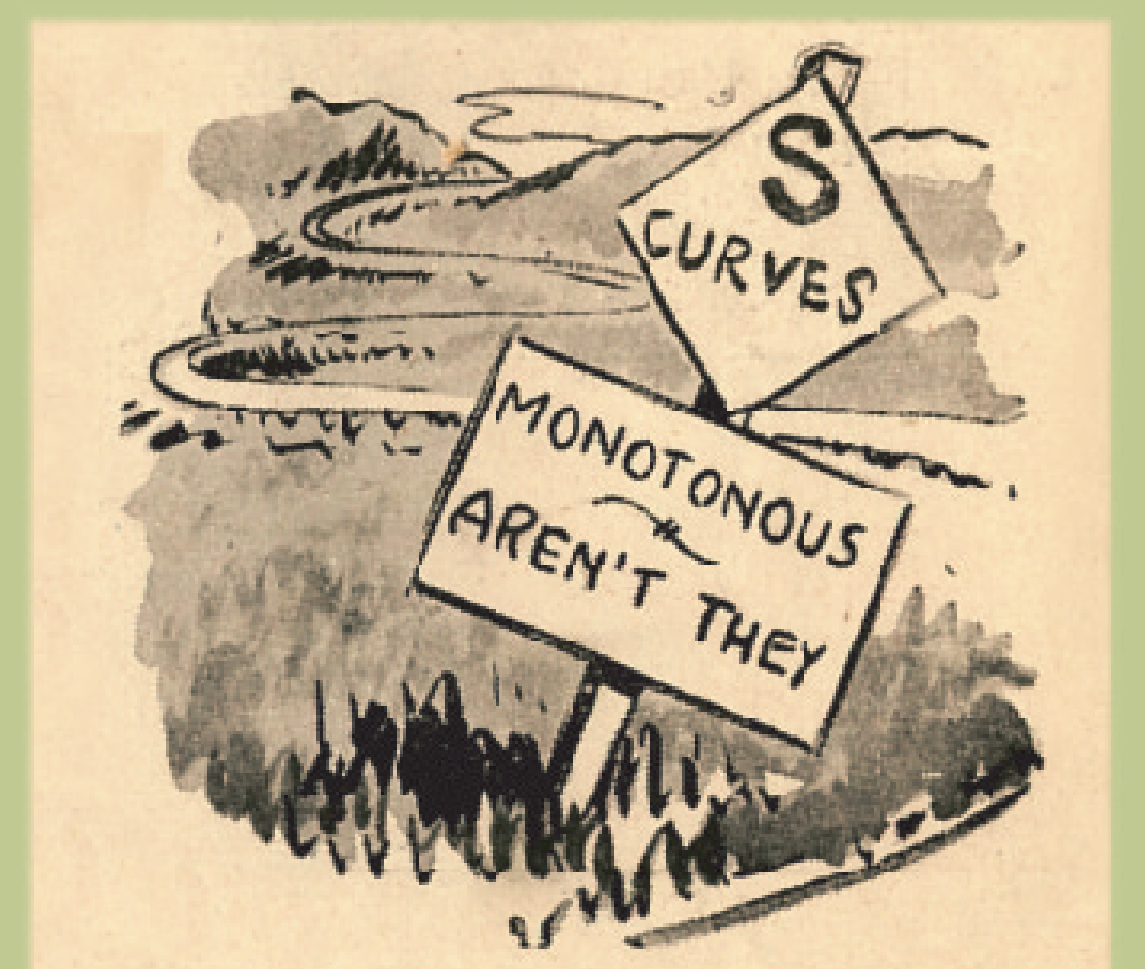
CURVE A ESSE MONOTONE, VERO?
